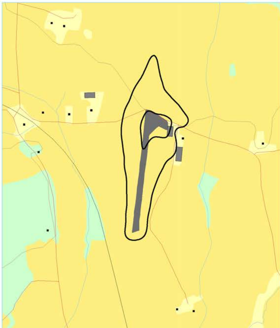
Figur 9-1. L_{den} 52 og 62 dBA for omsøkt situasjon. Målestokk 1:10 000.
